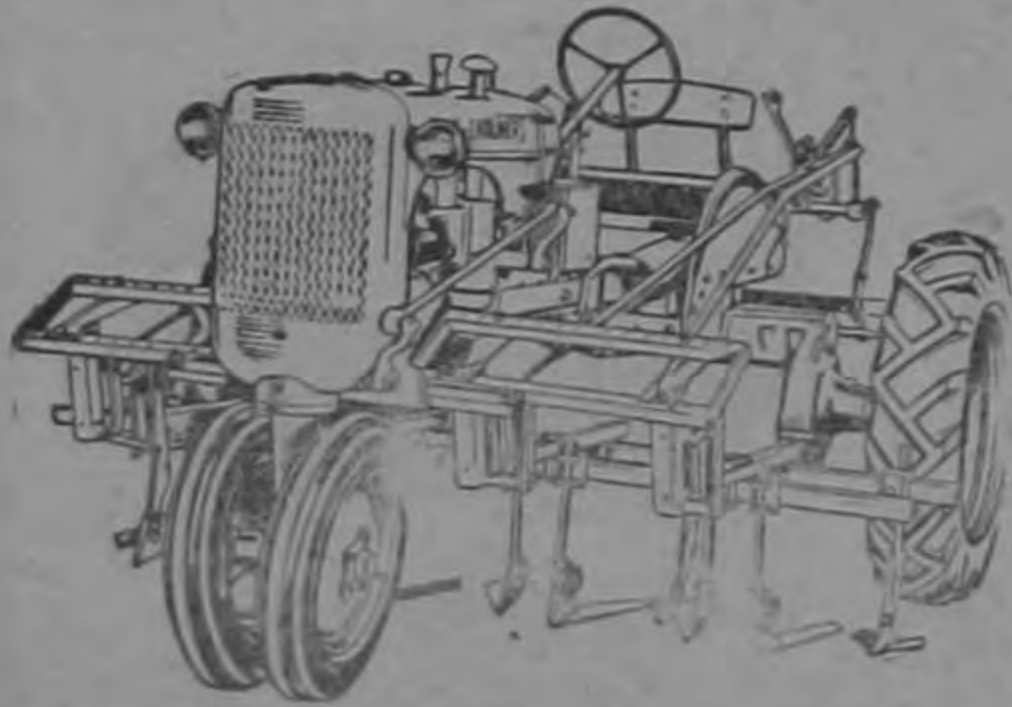
TRACTOR "C" con CULTIVADORA
